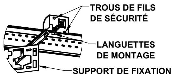
FIGURE 3 PLAFONDS SUSPENDUS
