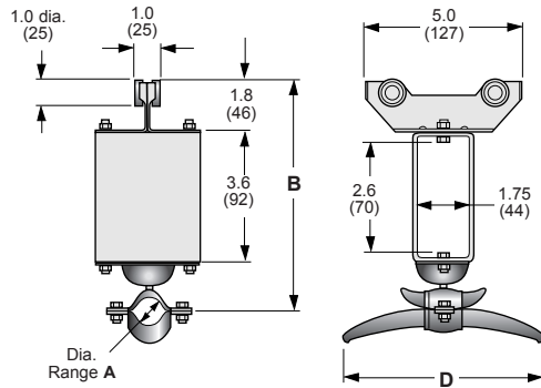
TOW ARM CTA-01 Wgt: 3.00 lbs
