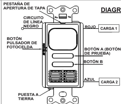
FIGURA 1 – MULTI-TECH, CIRCUITO DOBLE, PUESTA A TIERRA
