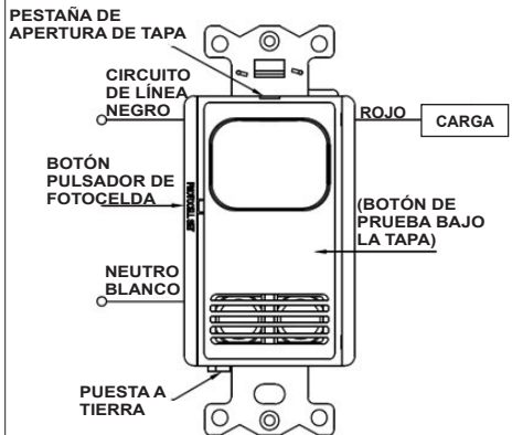
FIGURA 4 – INFRARROJO PASIVO, CIRCUITO SENCILLO, SIN BOTÓN, CONEXIÓN NEUTRA
