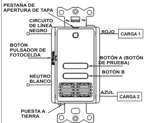
FIGURA 3 – ULTRASÓNICO, CIRCUITO DOBLE, CONEXIÓN NEUTRA
