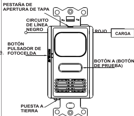
FIGURA 2 – MULTI-TECH, CIRCUITO SENCILLO, PUESTA A TIERRA
