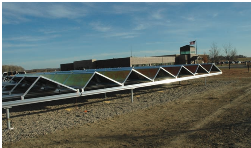
Contratista presupuesto 7 días con una cuadrilla de dos para la instalación de los pilotes helicoidales. El sistema completo fue instalado en dos días.
