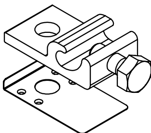
WEEB-LUG-8.0
