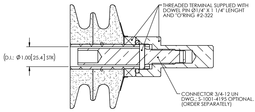
SECTION A-A SCALE 1 : 3
