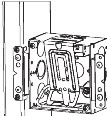
Step 2. Remove Pry-Out(s).
