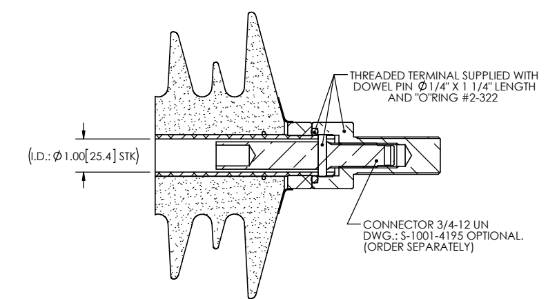
SECTION B-B SCALE 1 : 4
