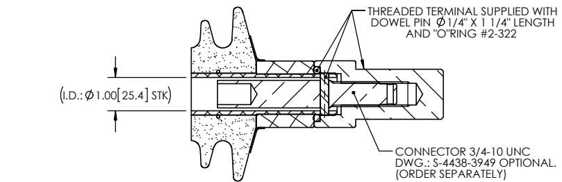
SECTION A-A SCALE 1 : 4
