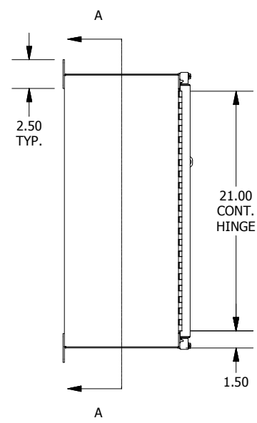
LEFT SIDE
