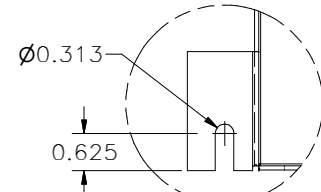
DETAIL D (2 PL.)
