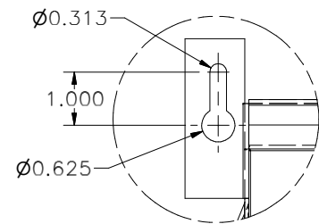
DETAIL C (2 PL.)
