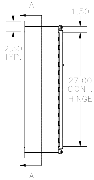
LEFT SIDE
