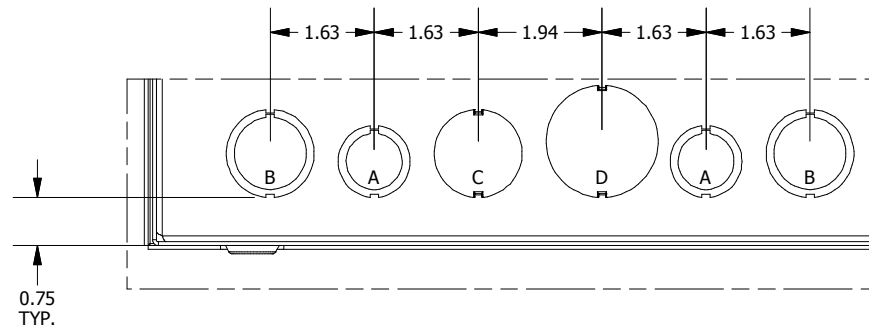
DETAIL B (3 PL.) (K.O. PATTERN)
