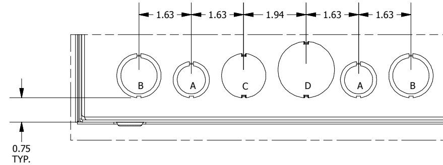
DETAIL B (4 PL.) (K.O. PATTERN)
