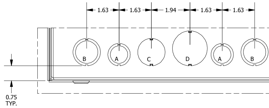
DETAIL B (4 PL.) (K.O. PATTERN)
