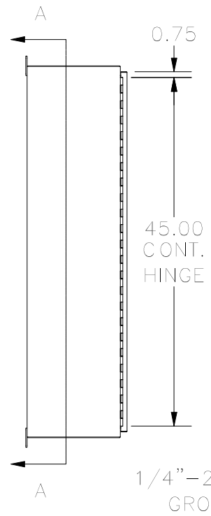
LEFT SIDE
