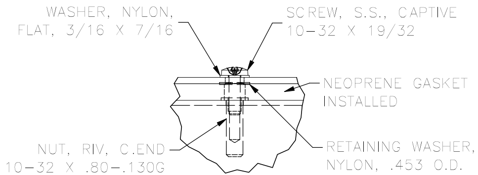
DETAIL D (6 PL.)
