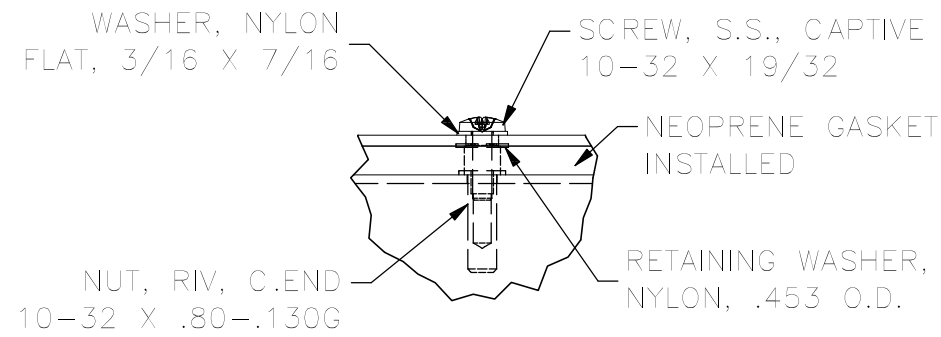
DETAIL D (8 PL.)
