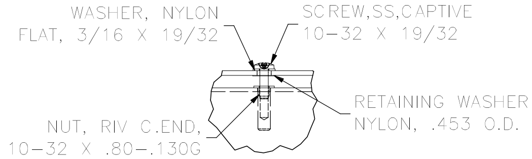
DETAIL D (12 PL.)
