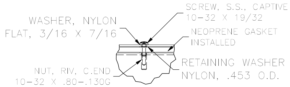
DETAIL D (20 PL.)
