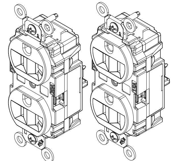
CATALOG NO: HBL8300ST (NOT SHOWN TO SCALE)
