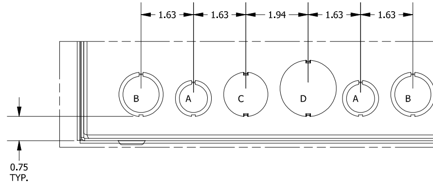
DETAIL B (4 PL.) (K.O. PATTERN)
