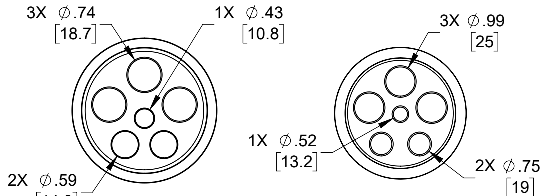
CAT. # 2408 SCALE 1 : 3
