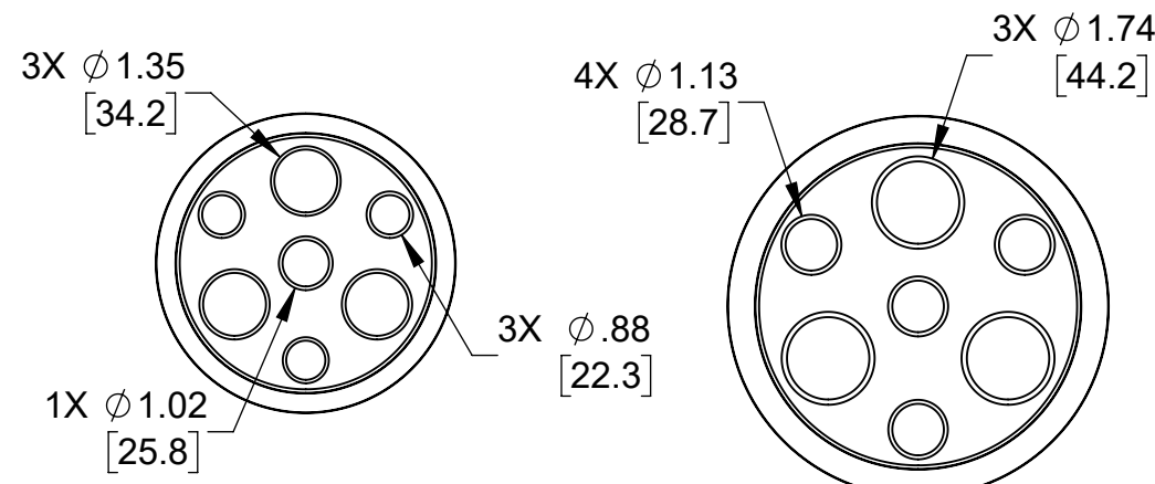
CAT. # 2410 SCALE 1 : 4
