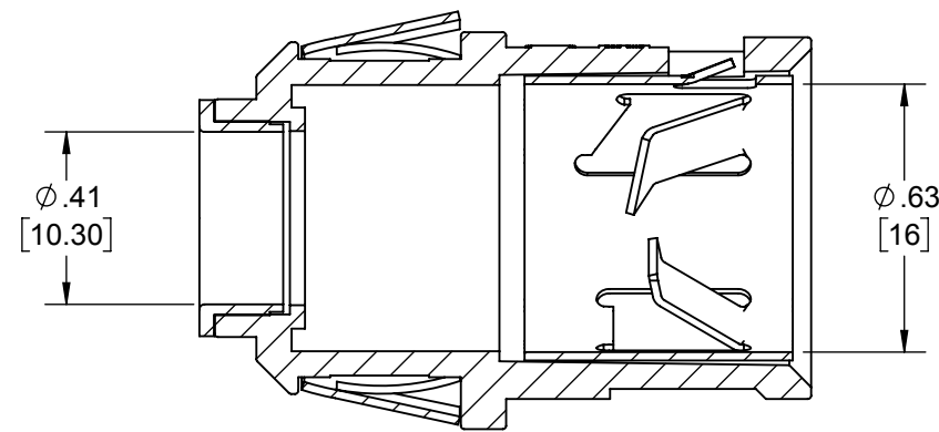
SECTION A-A SCALE 2 : 1
