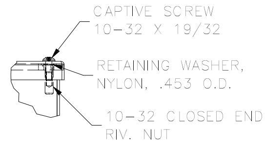
DETAIL N (2 PL.)
