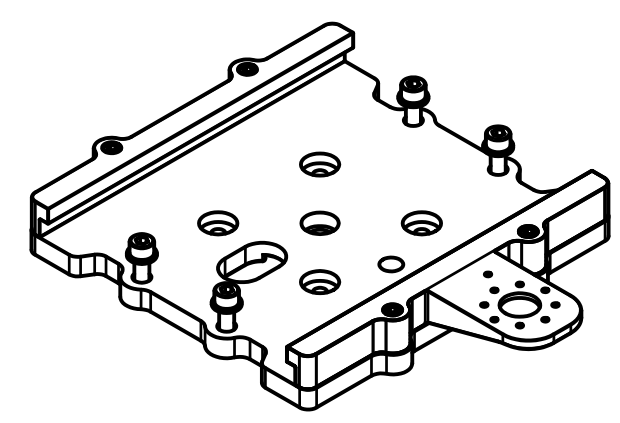
HBLIMBJ (1/4 SCALE)
