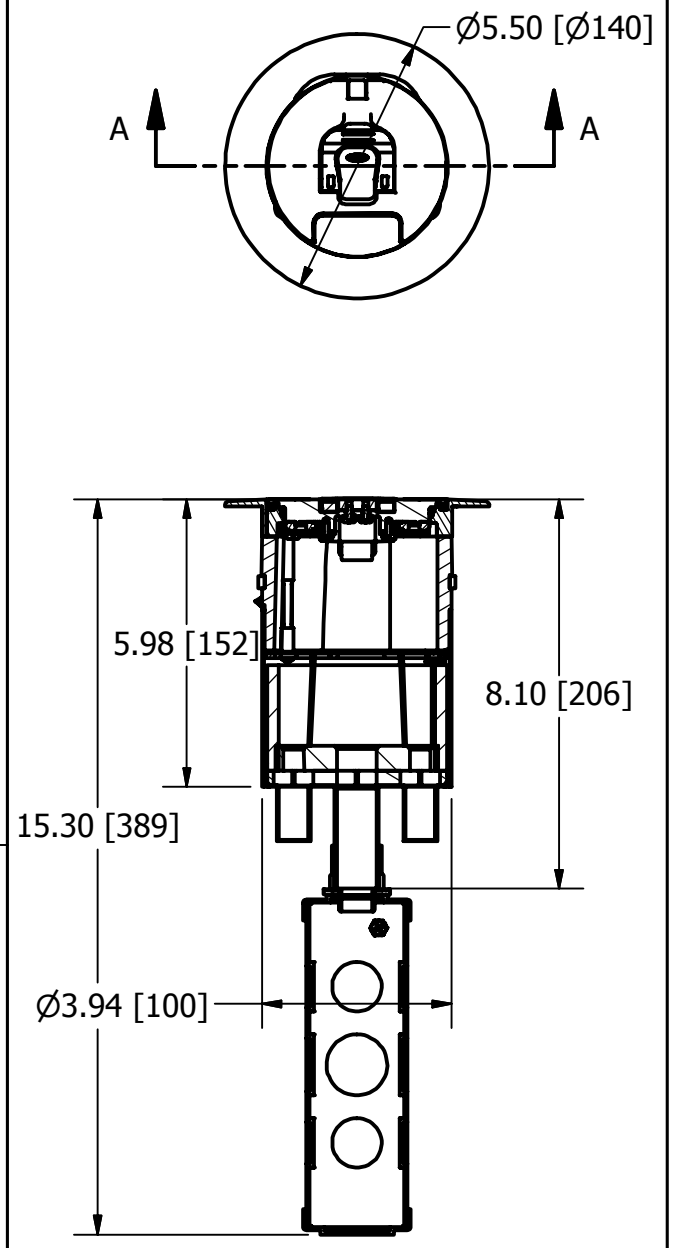
SECTION A-A
