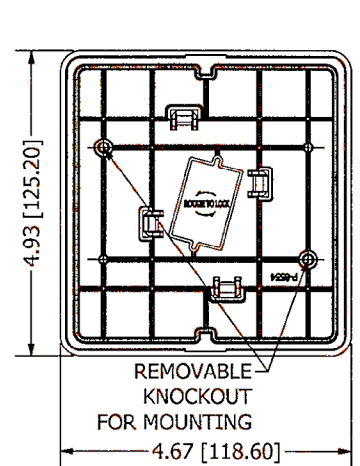
BOTTOM
