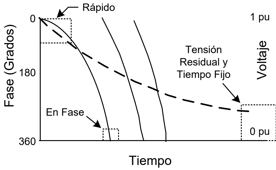
Figura 3 Métodos de Transferencia con Transición Abierta
