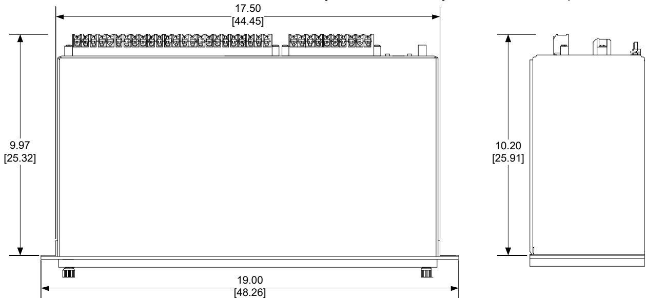
Figura 9 Dimensiones para Montaje Vertical
