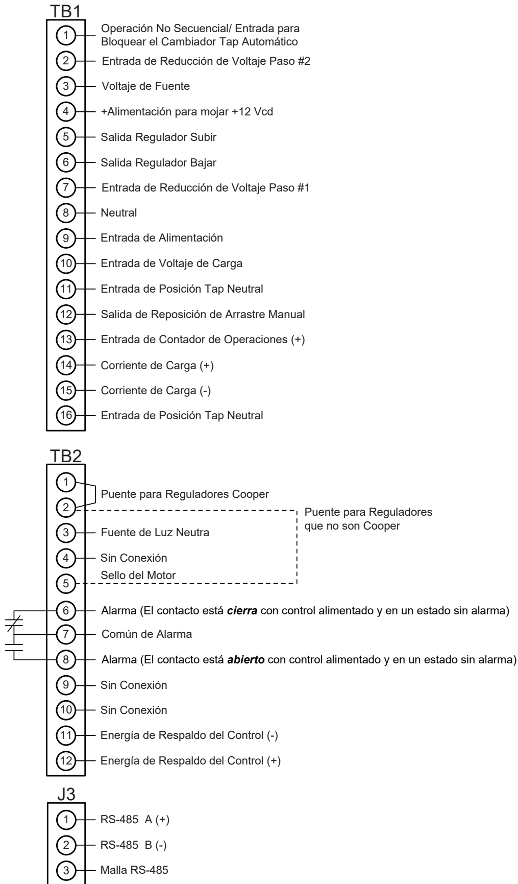
Figura 7 Conexiones Típicas Externas del M-6200A
