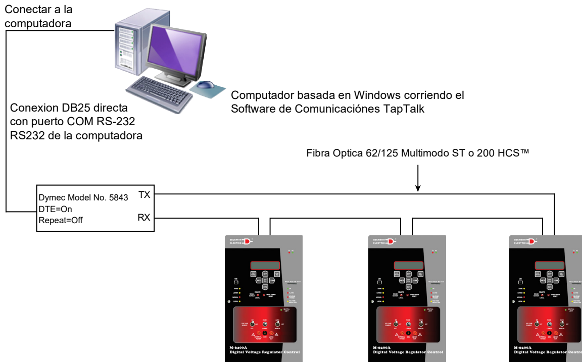
Figura 2 Lazo de Conexión de Fibra Óptica
