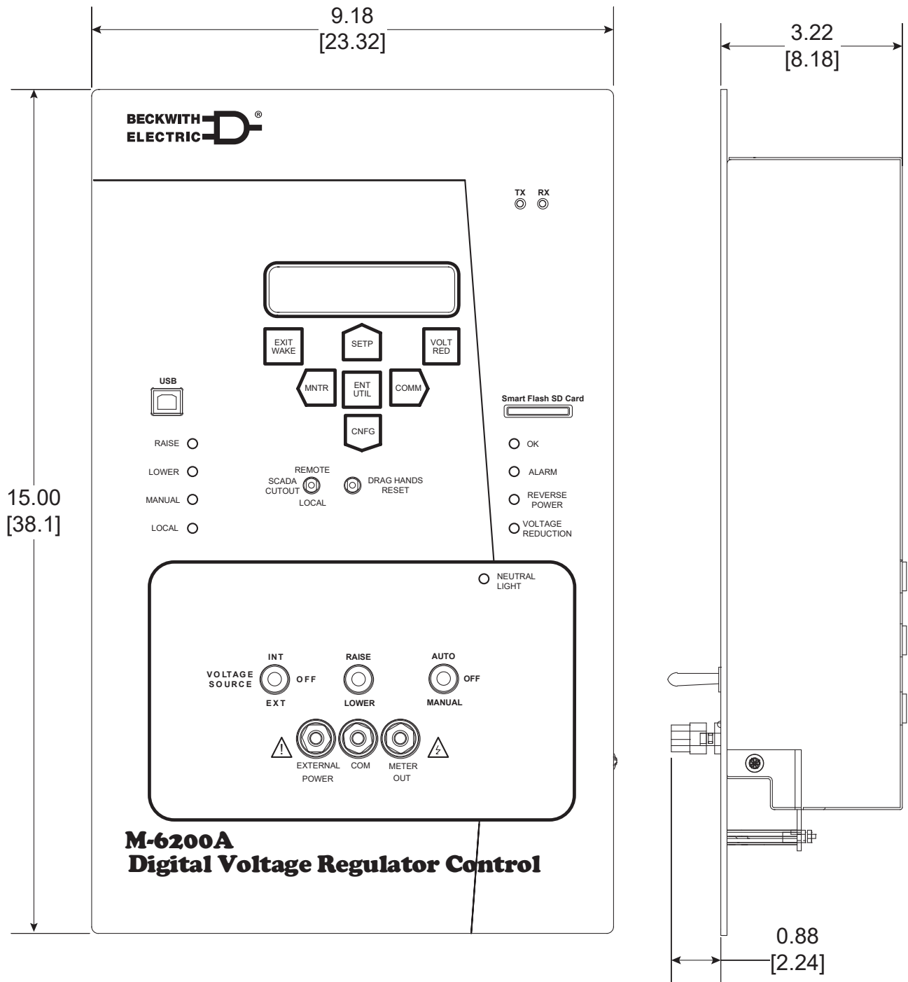
Figura 6 Dimensiones de contorno del M-6200A
