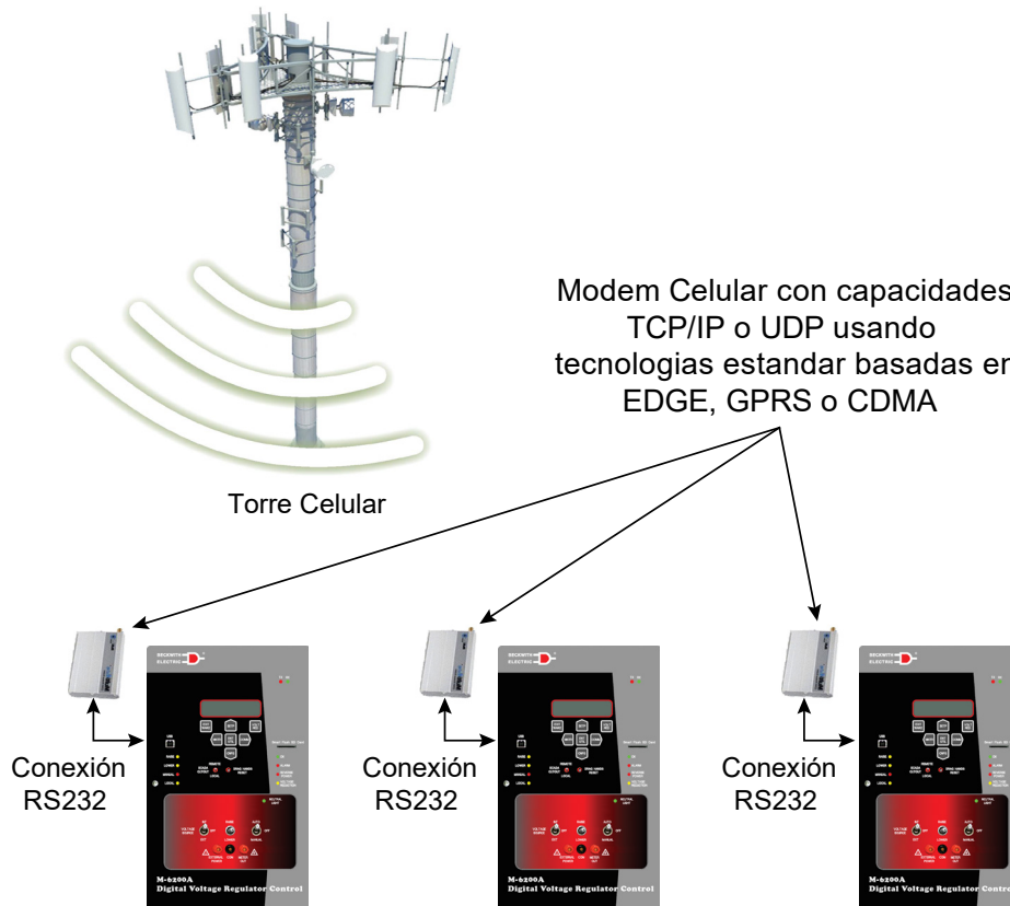
Figura 5 Red de Modem Celular Ambiental
