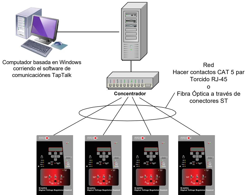
Figura 4 Conexión de Red Opcional Ethernet
