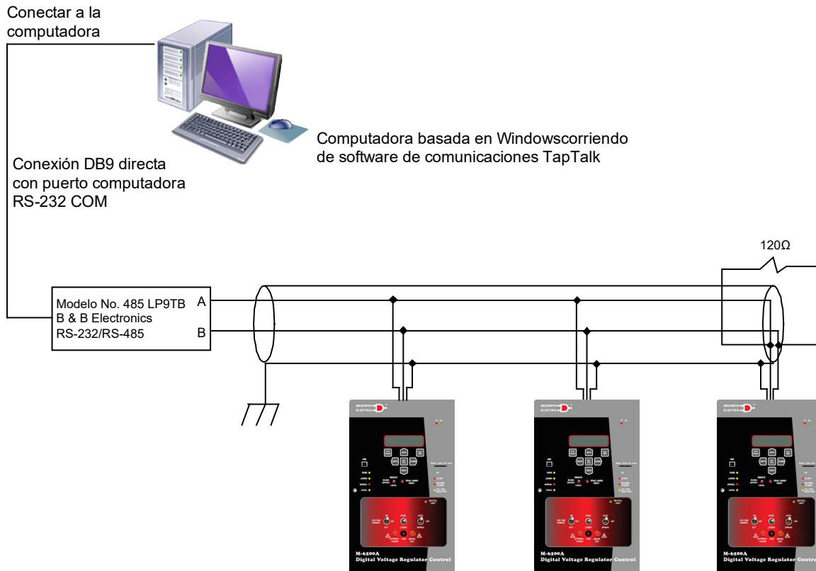
Figura 3 Conexión de red RS-485
