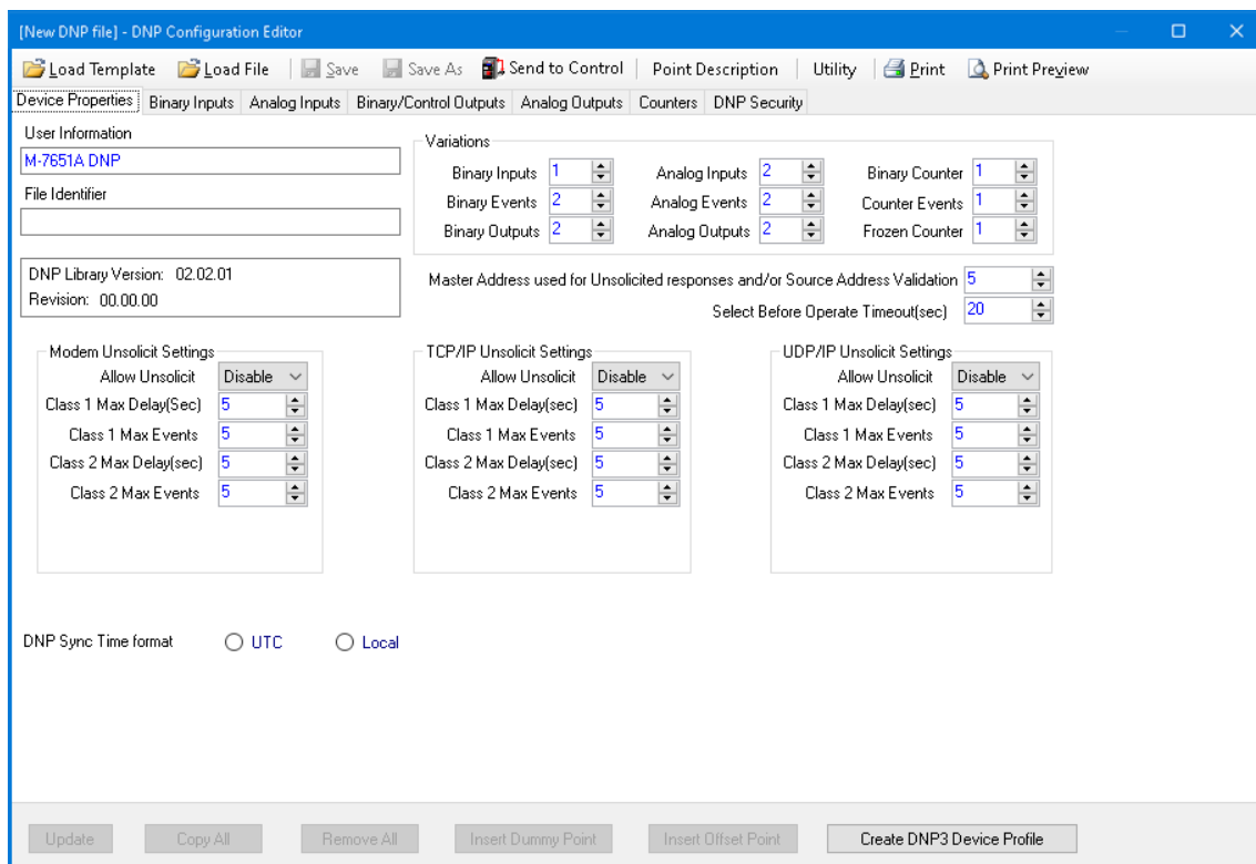
Figura 1-1 Pantalla de editor de configuración DNP
