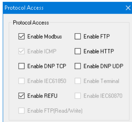
Figura 2-3 Pantalla de Seguridad de Puerto de Comunicaciones/Protocolo de Acceso
